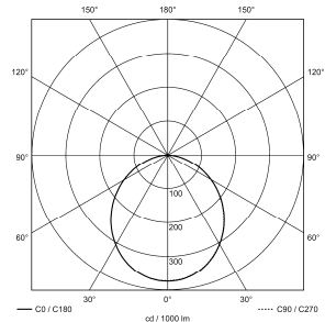
配光曲線
