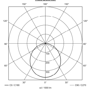
配光曲線
